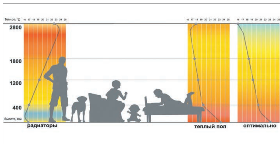
Рис. 1. Графики распределения температуры по высоте помещения
