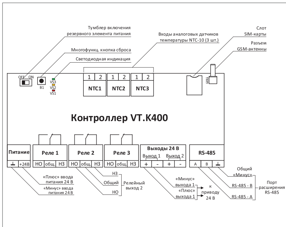
Рис. 24. Назначение контактов и элементов управления VT.K400
