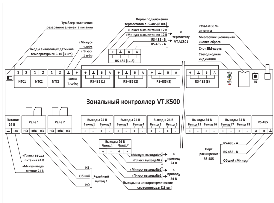
Рис. 26. Назначение контактов и элементов управления VT.K500
