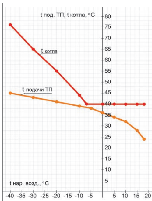
Рис. 29. Погодозависимые графики котла и насосно-смесительного узла.
