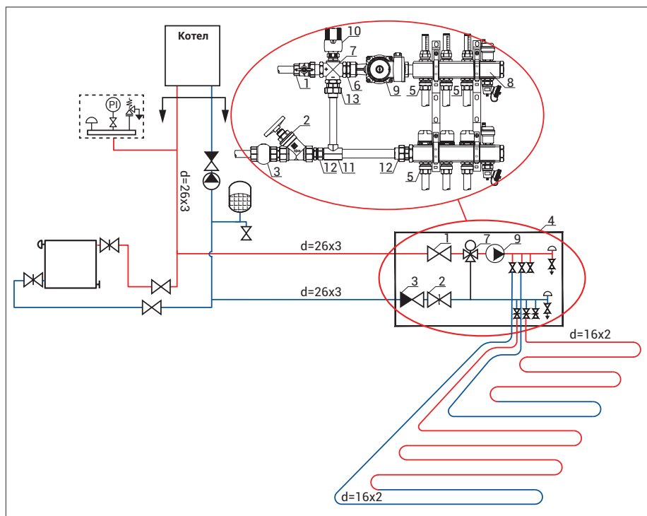
Схема комбинированного отопления помещений (водяной теплый пол и радиаторы). Площадь водяного теплого пола до 80 м² .
