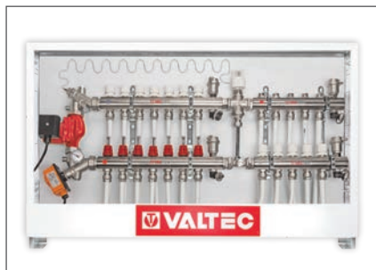
Комбинированная система на базе узла VT.DUAL
