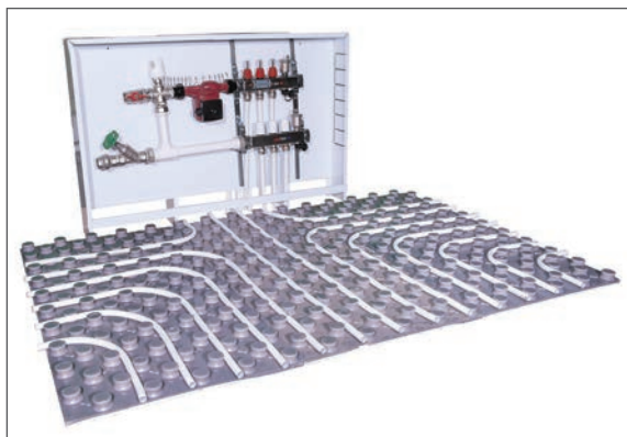
Схема комбинированного отопления помещений (водяной теплый пол и радиаторы). Площадь водяного теплого пола до 80 м² .
