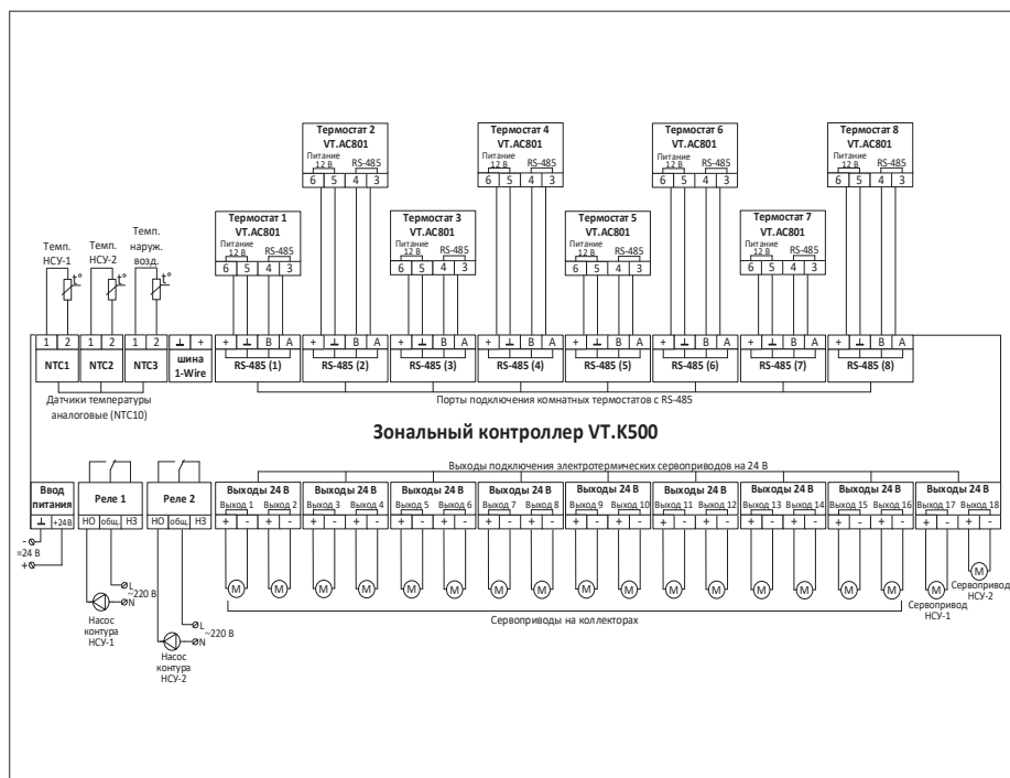
Рис. 27. Назначение контактов и элементов управления VT.K500
