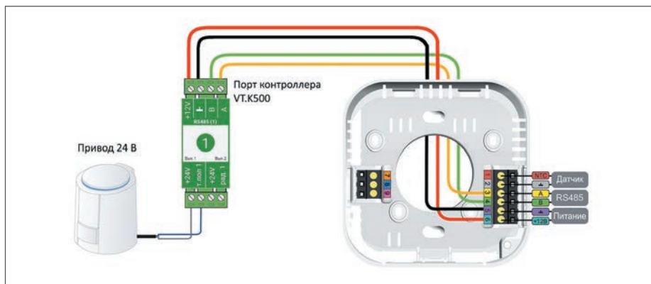
Рис. 33. Схема подключения термостата и привода при работе с зональным контроллером VT.K500
