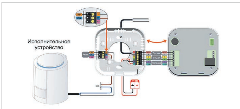
Рис. 32. Схема подключения НЗ привода при автономной работе термостата
