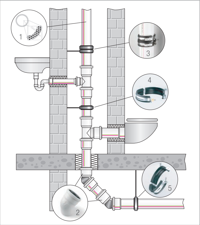
Рис. 4-1 Минимизация шума
