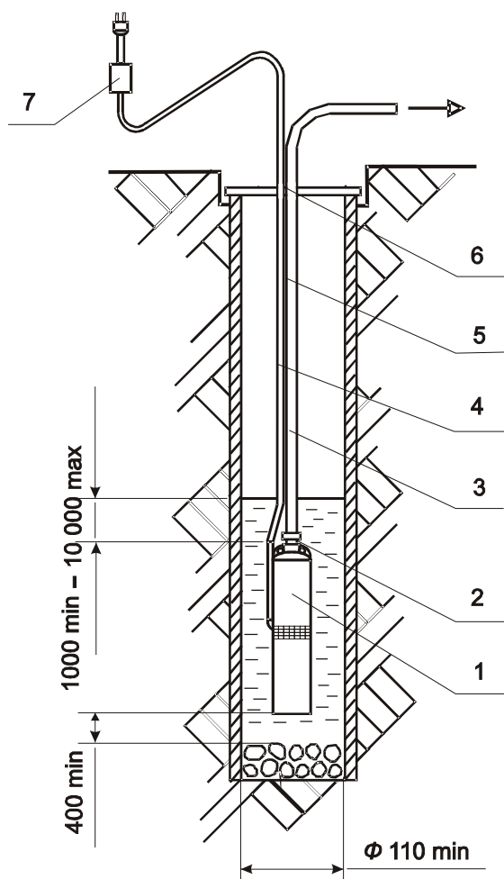
Рис 4. Схема установки электронасоса БЦПЭ в скважину (размеры в мм). 1 - электронасос; 2 - хомут трубопровода; 3 - трубопровод; 4 - шнур сетевого питания; 5 - трос; 6 - место крепления подвески; 7 - коробка конденсаторная.
