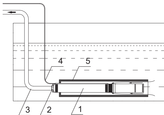
Рис 4. Схема установки электронасоса БЦПЭ в скважину (размеры в мм). 1 - электронасос; 2 - хомут трубопровода; 3 - трубопровод; 4 - шнур сетевого питания; 5 - трос; 6 - место крепления подвески; 7 - коробка конденсаторная.
