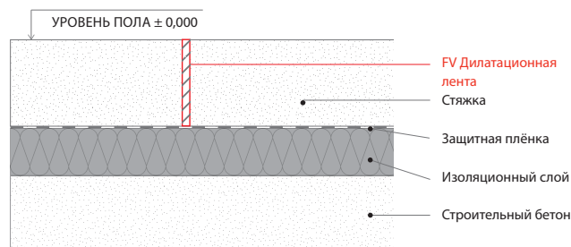
Рисунок 5: Деформационный шов стяжки при кладке твёрдых покрытий пола (плитка, каменный пол, ламинат)
