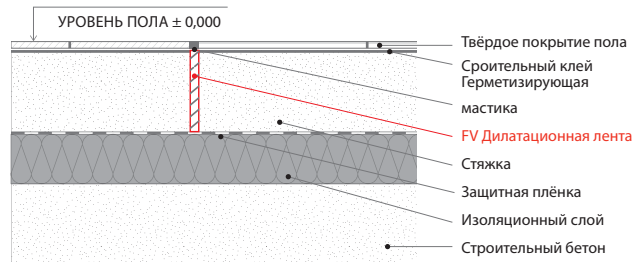
Рисунок 6: Деформационный шов стяжки с отделяющим слоем при кладке твёрдых покрытий пола (плитка, каменный пол, ламинат)
