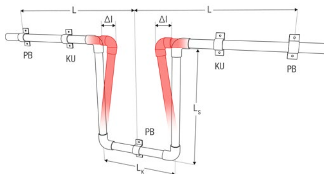
РИС.5 „U“ - компенсатор
