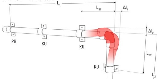
РИС 3 .. L " - компенсатор
