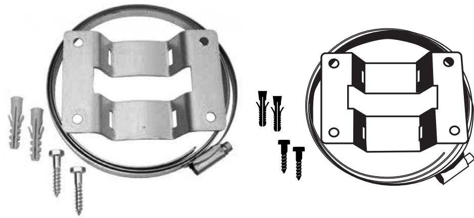
Хомутное крепление для расширительного бака
