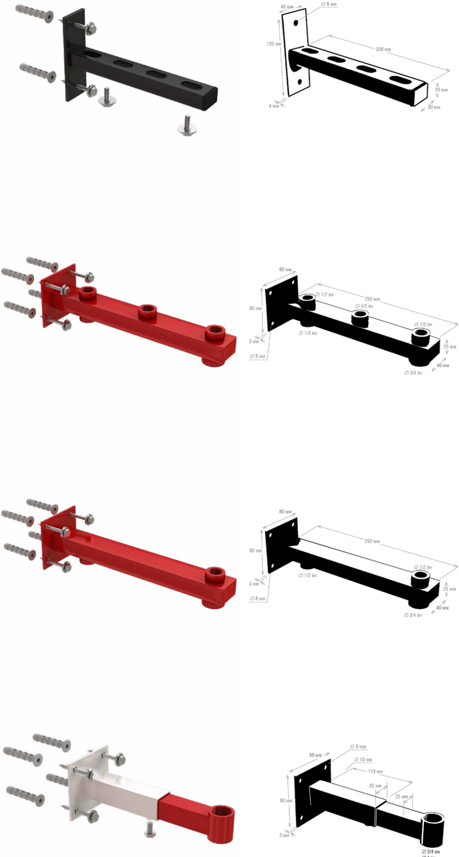
Крепление для коллектора
