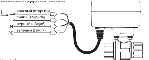
Рис. 3 Электрическая схема подключения крана с электроприводом серии Neptun PROFIS 230B
