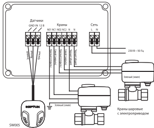
Рис. 3. Схема подключения датчиков контроля протечек и кранов шаровых с электроприводом к модулю управления
