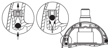
Рис. 14 Автоматическое удаление воздуха
