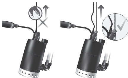
Рис. 3 Перемещение насоса
