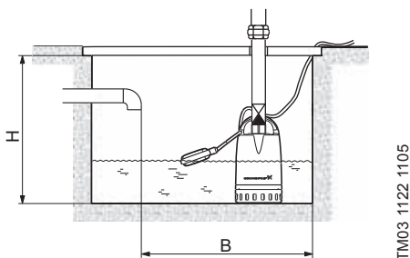
Рис. 4 Минимальные монтажные размеры
