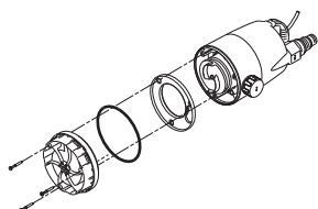
Рис. 17 Демонтаж деталей, находящихся в днище насоса
