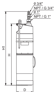
Рис. 11 Модель SBA со встроенным сетчатым фильтром
