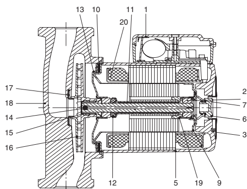
Рис. 29 Модель насоса UPS 25-120
