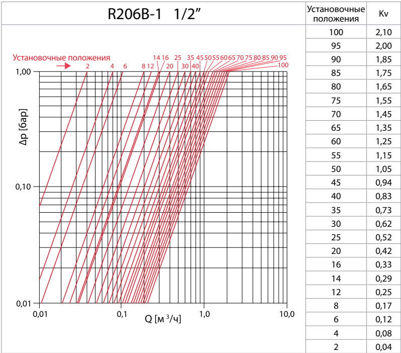
Рис. 4. Диаграмма значений предварительной настройки клапана.
