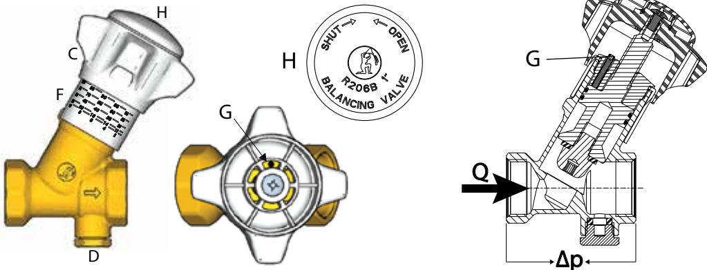
Рис. 3. C – рукоятка, D – штуцер для импульсной трубки или слива (1/4" внутр. резьба), F – шкала для установки 0% ÷ 100% (25 положений), G – винт блокировки (ограничивает ход рукоятки), H – съёмная крышка рукоятки (для блокировки).
